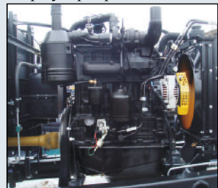
Дизельный двигатель Д-245.5 мощностью 65 кВт
